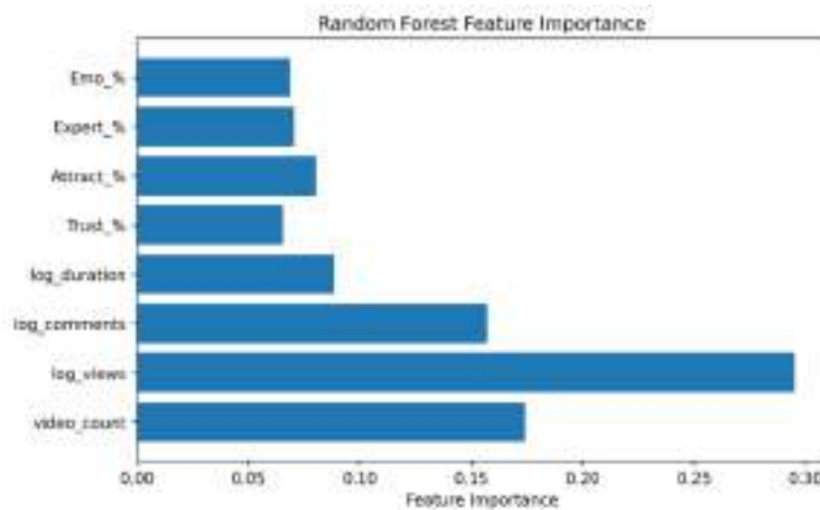
ภาพที่ 2 คุณลักษณะสำคัญ (Feature Importance) ของแบบจำลองการสุ่มป่าไม้ (Random Forest)
